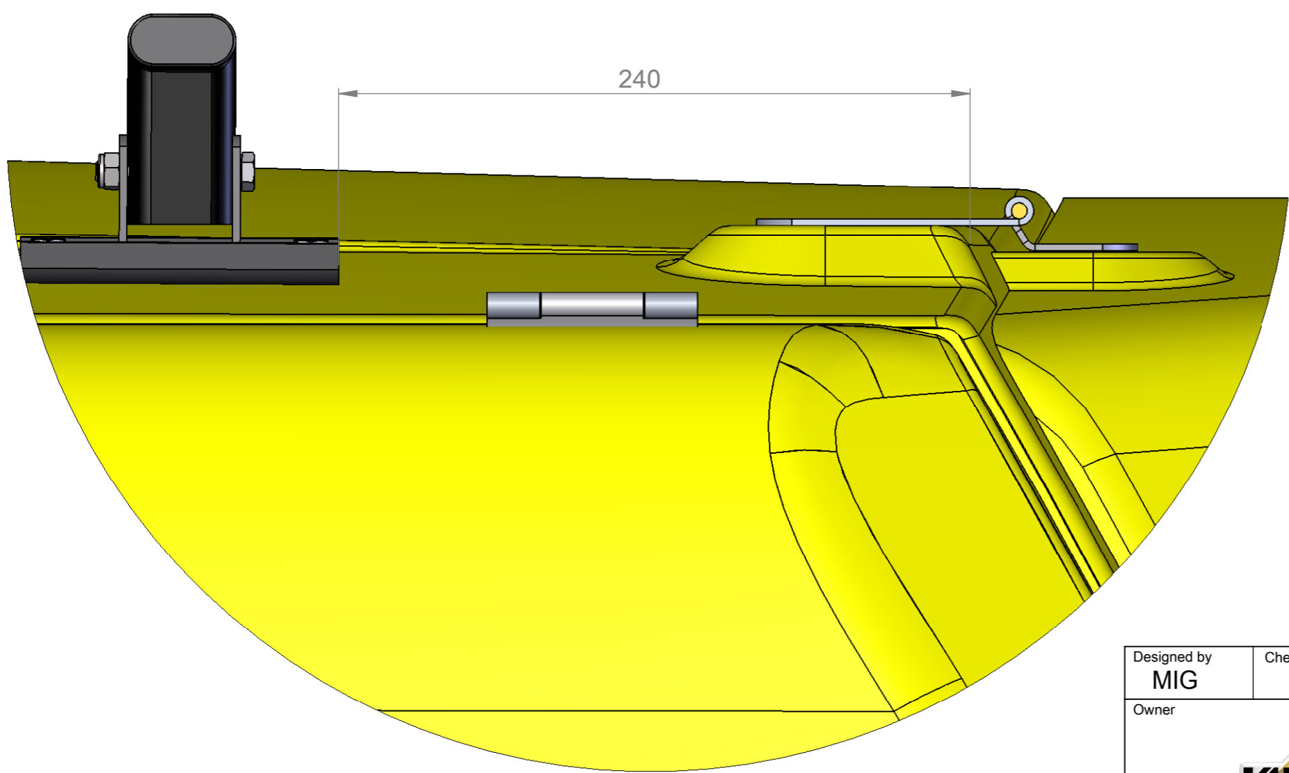
A (1 : 2)
